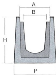
PIANTA canale con bordo zincato
